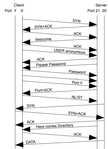
FTP Sitzung
