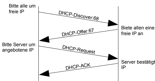
DHCP
