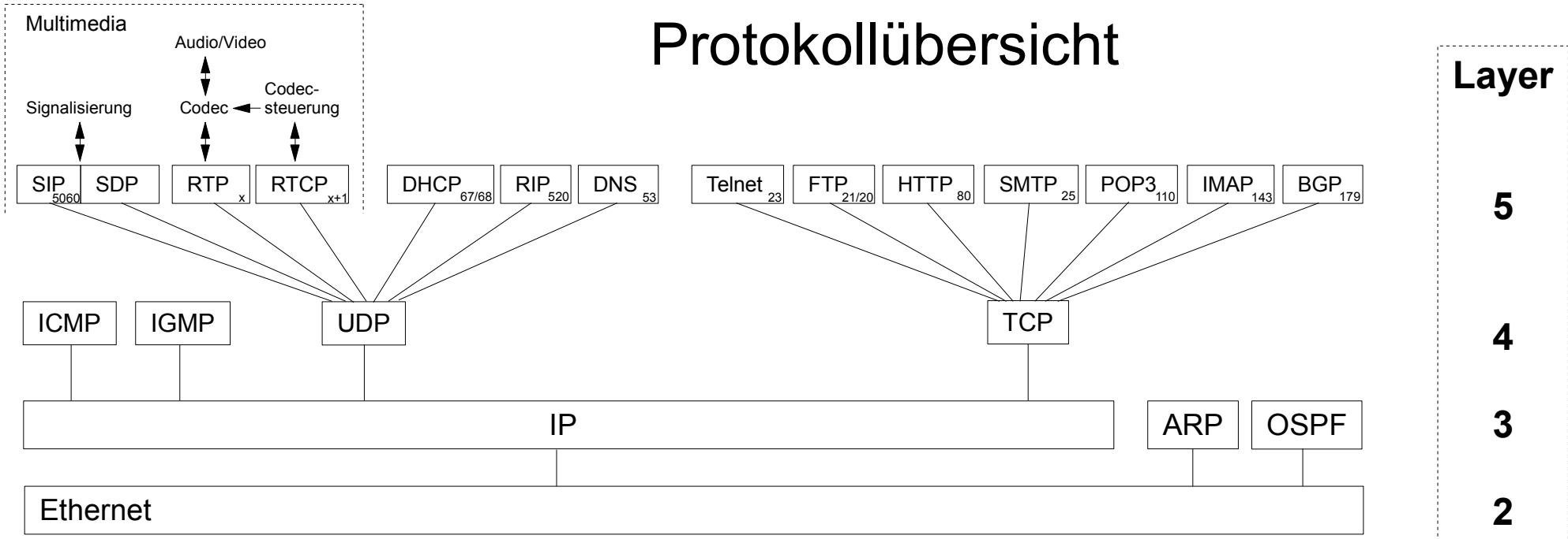
ARP
