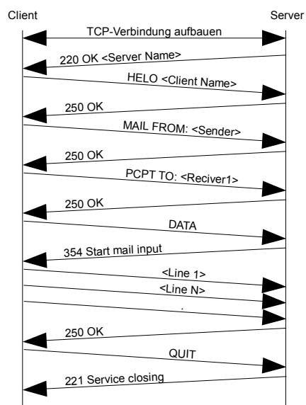
SMTP Sitzung
