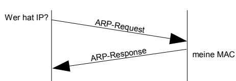
ARP
