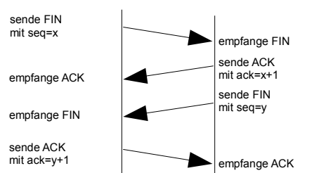
TCP Verbindungsabbau
